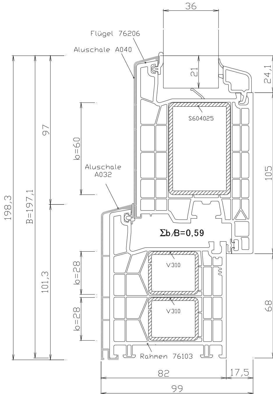
Bild 3: Profilquerschnitt Probekörper 06
