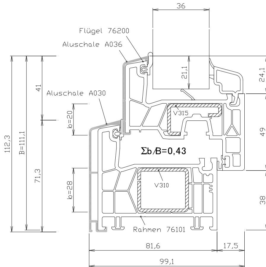
Bild 1: Profilquerschnitt Probekörper 04
