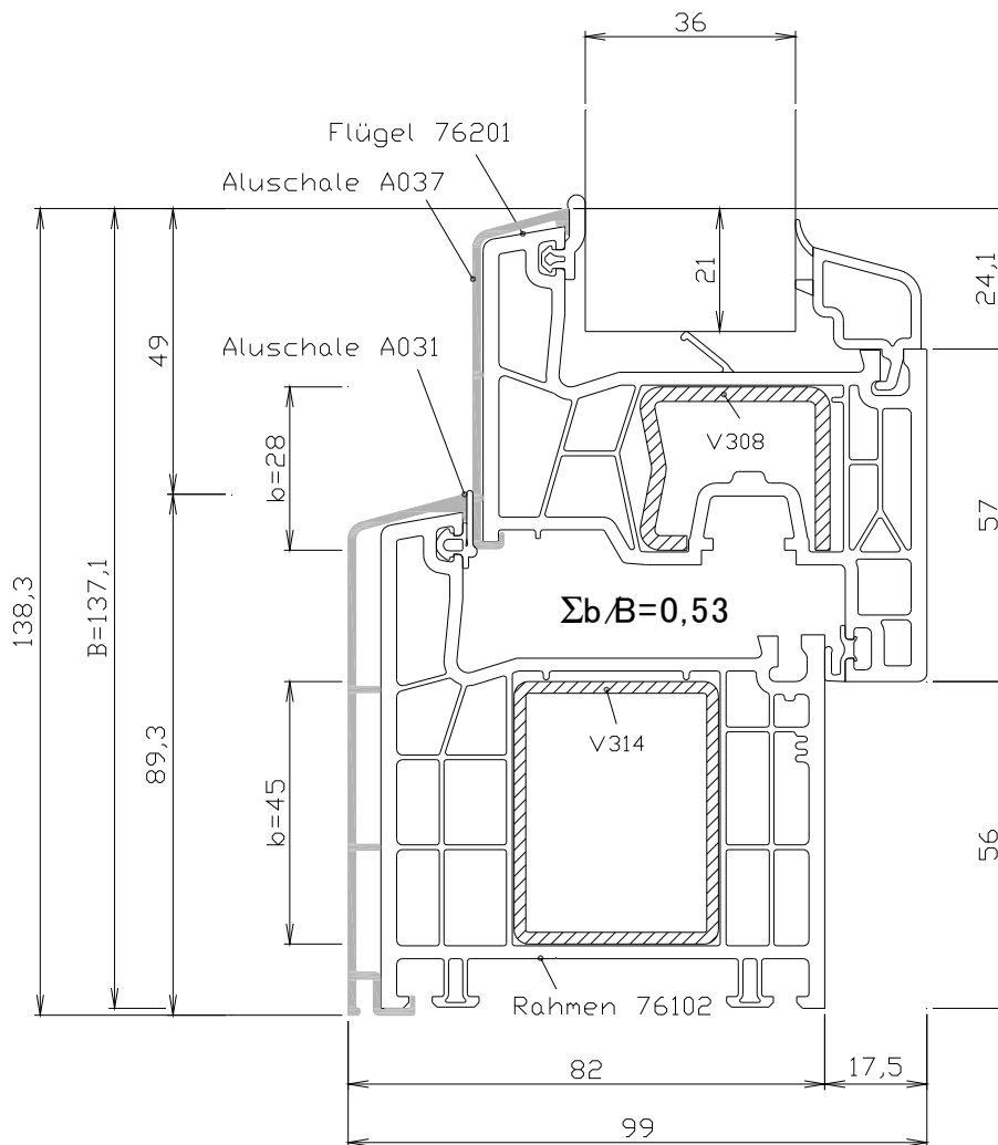
Bild 2: Profilquerschnitt Probekörper 05
